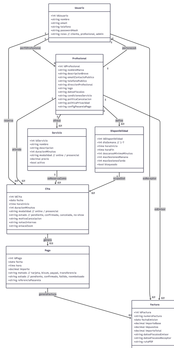
Fig. 2. Diagrama de clases preliminar del sistema. Versión ampliada disponible en este enlace de GitHub.
