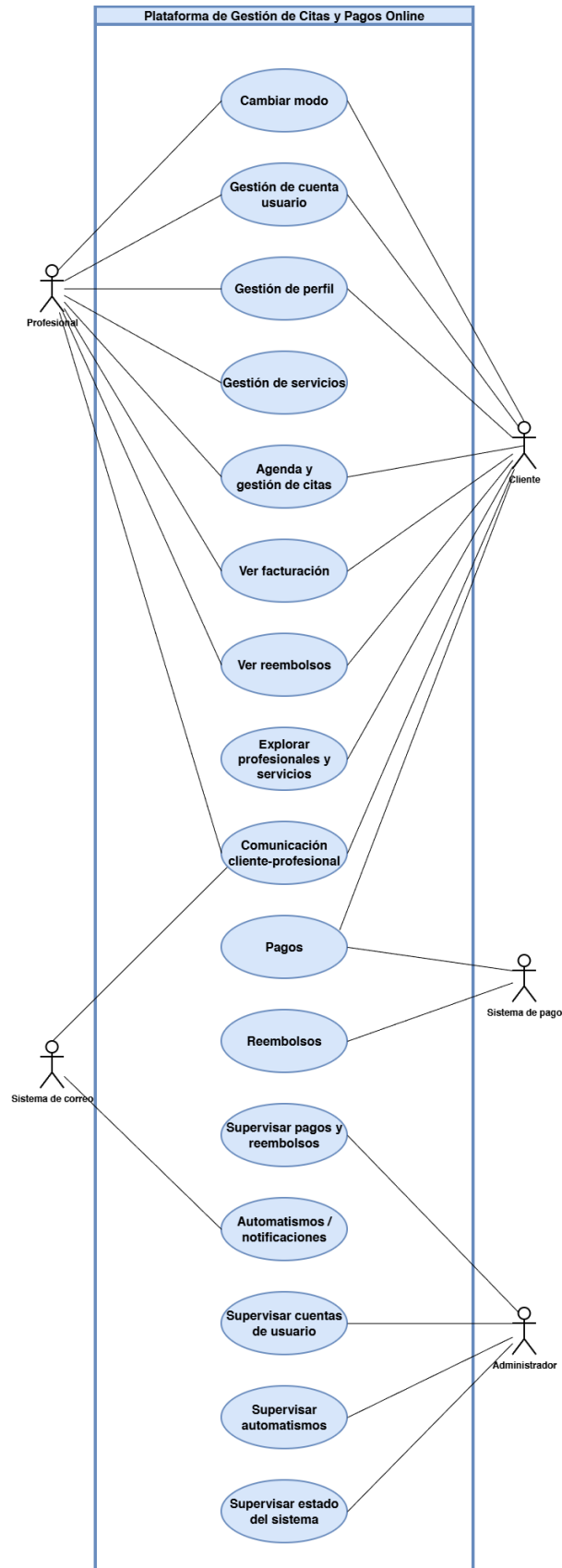
Fig. 1. Diagrama general de los casos de uso principales del sistema.
